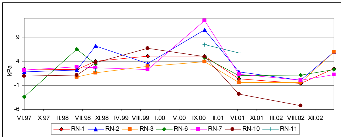
Obr. 1: Dlhodobé zmeny hodnôt povrchového reziduálneho napätia Fig. 1: Long-term changes of surface residual stress
